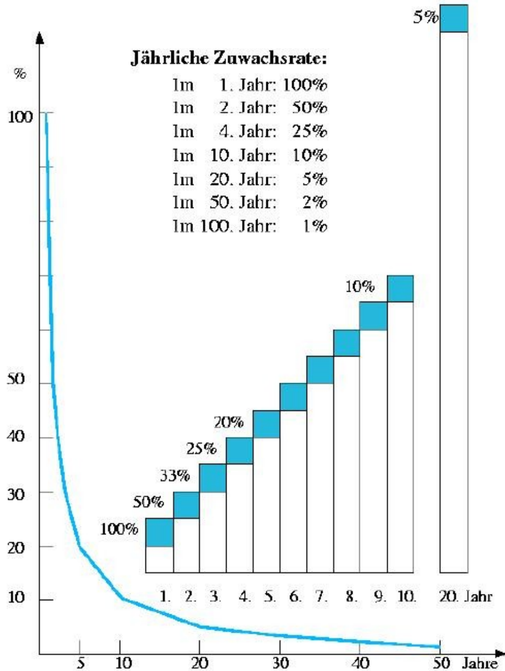
Abb. 2: Lineares Wirtschaftswachstum
